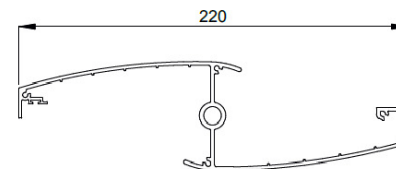
LAMELLEN - QUERSCHNITT
